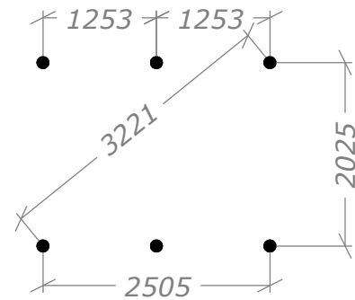
Runda plintar (1:50)
