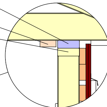
DETAIL D 1 : 10
